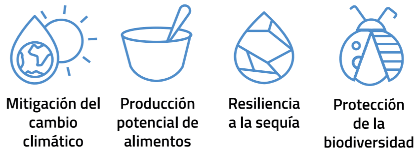
Figura 3: El papel fundamental del carbono orgánico del suelo (COS) para servicios esenciales derivados de los ecosistemas.
